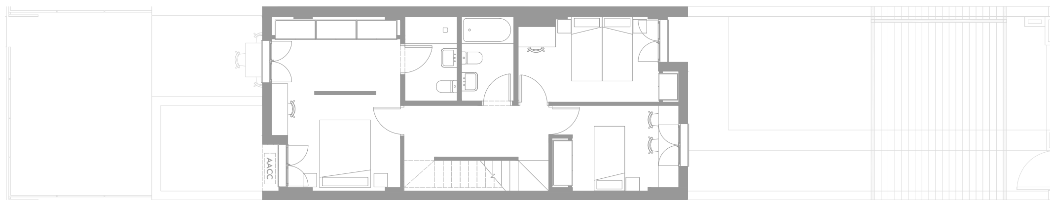
Planta primera
