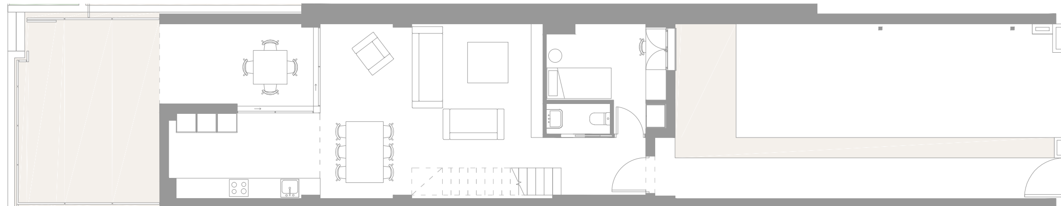
Planta baja
