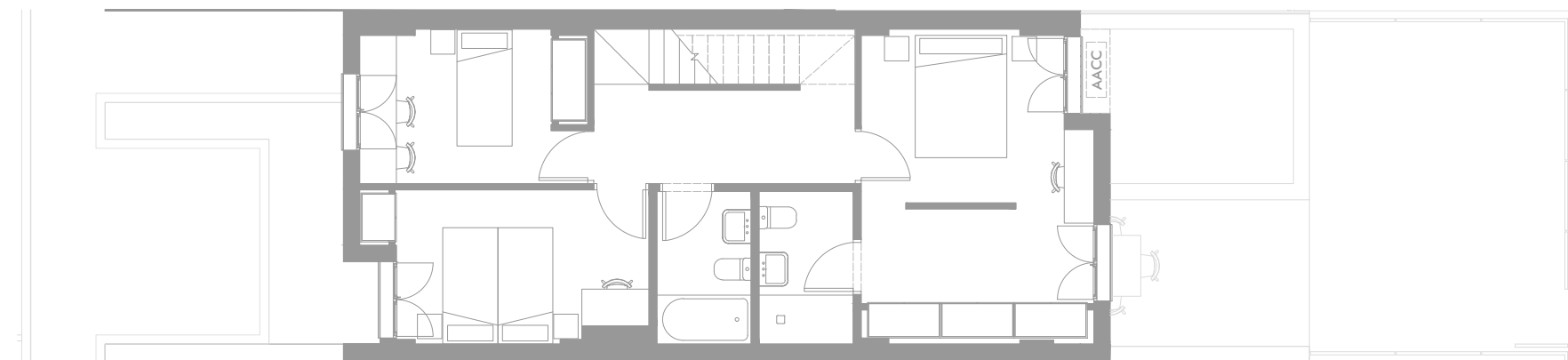
Planta primera
