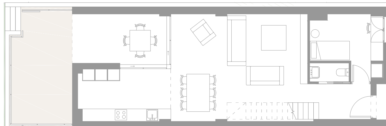
Planta baja
