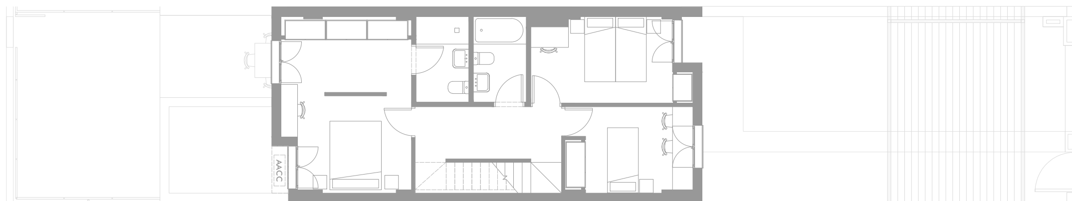
Planta primera
