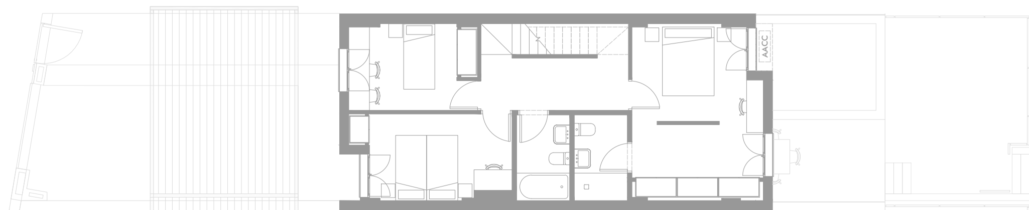
Planta primera
