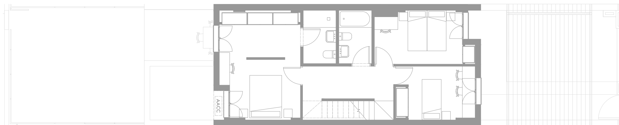
Planta primera
