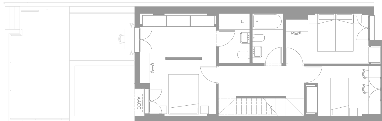
Planta primera
