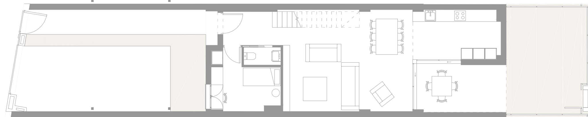
Planta baja
