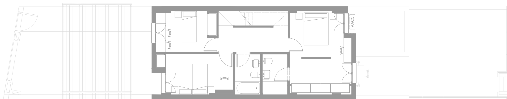
Planta primera
