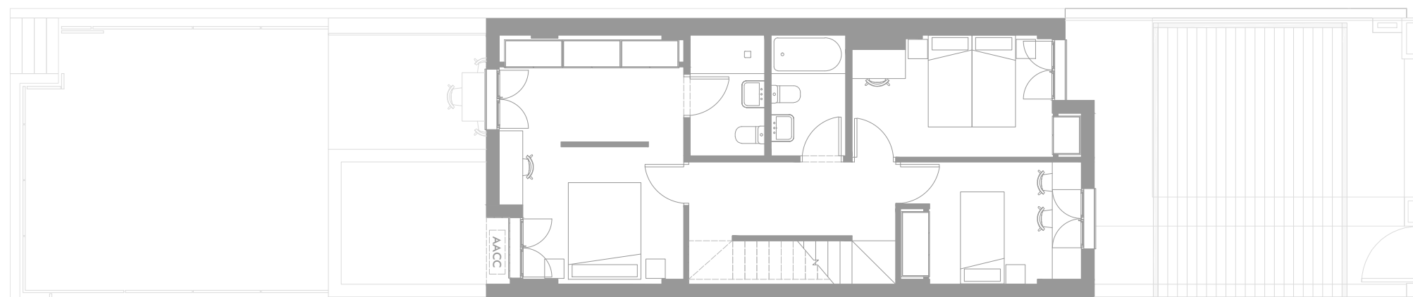
Planta primera
