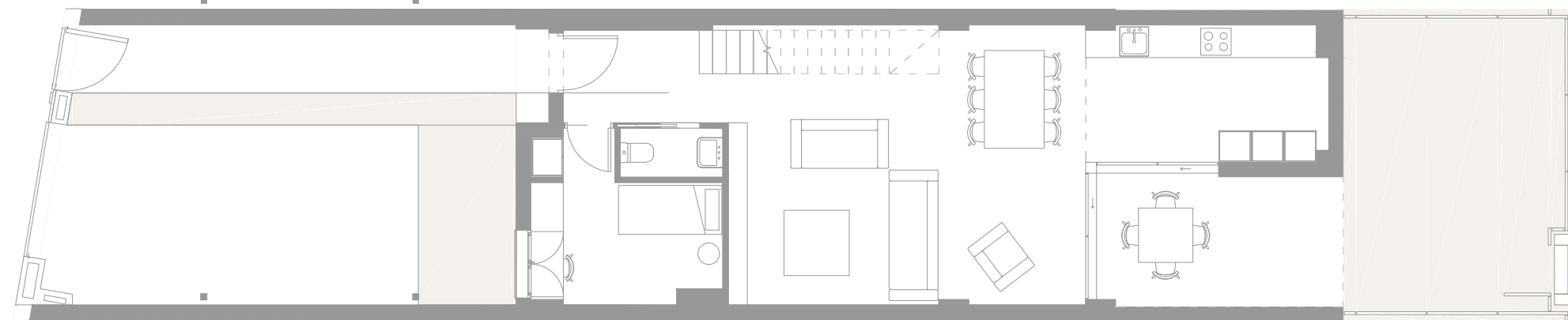
Planta baja
