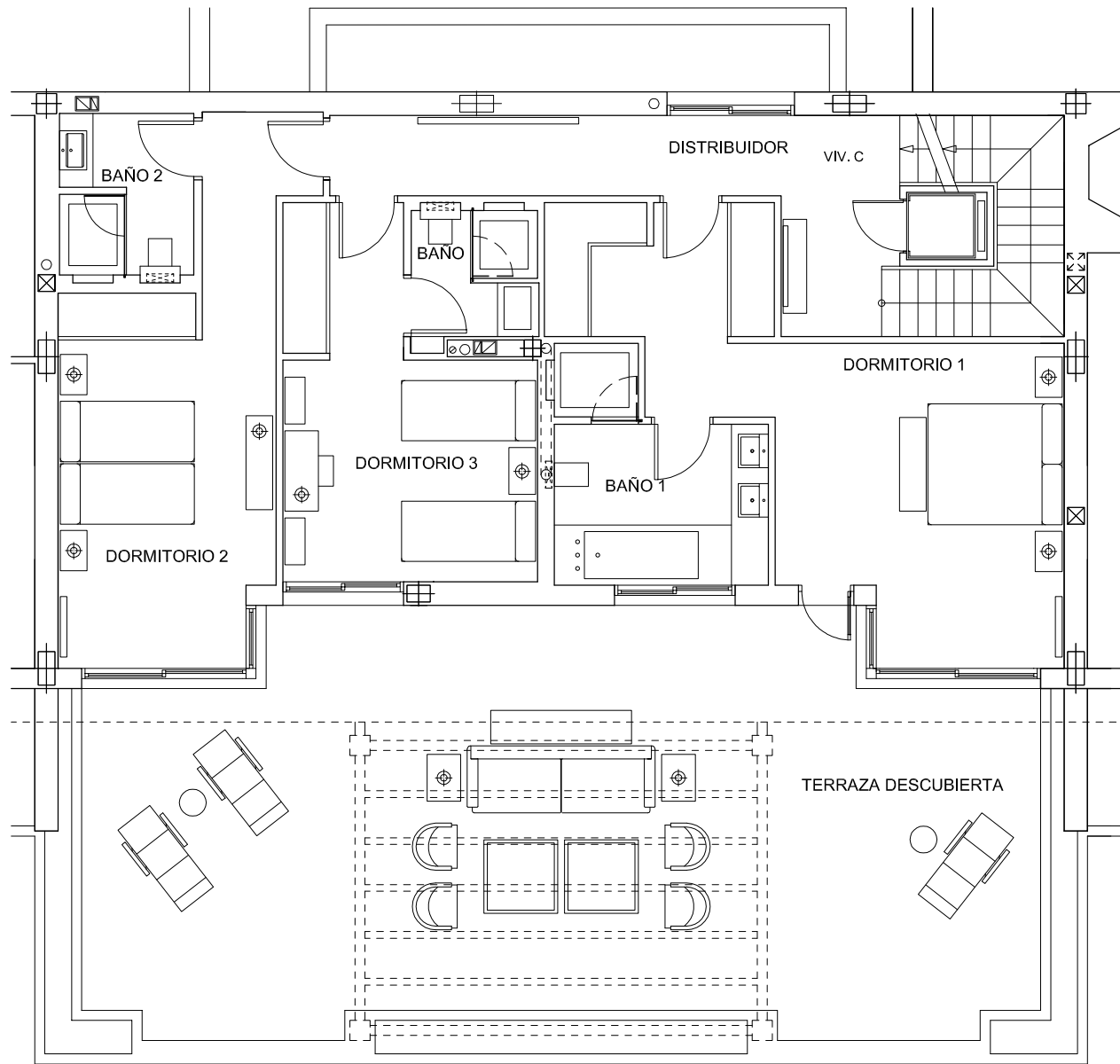
PLANTA ALTA
