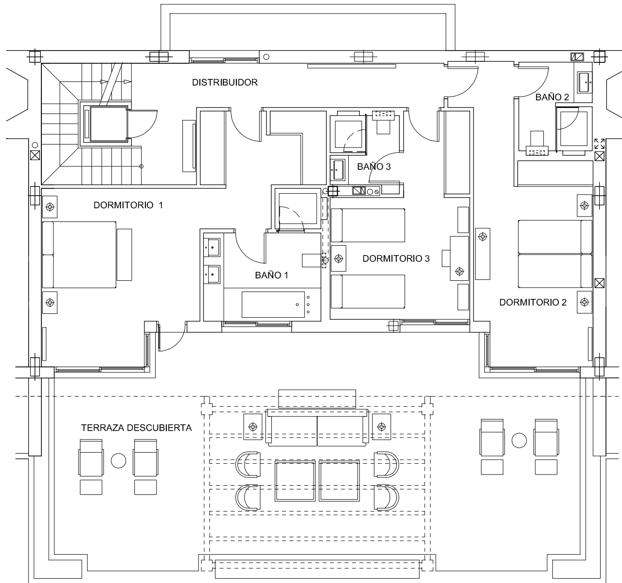
PLANTA ALTA
