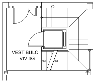
PLANTA BAJA
