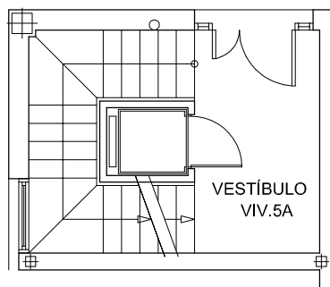
PLANTA BAJA
