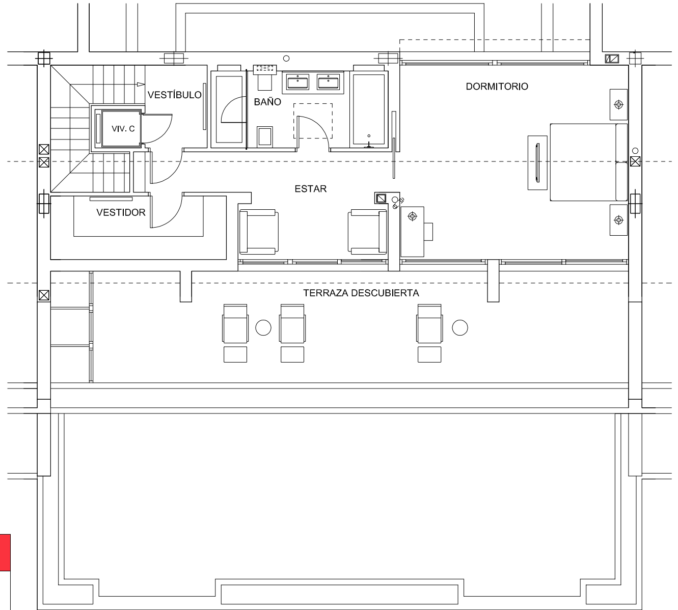
PLANTA SOLARIUM
