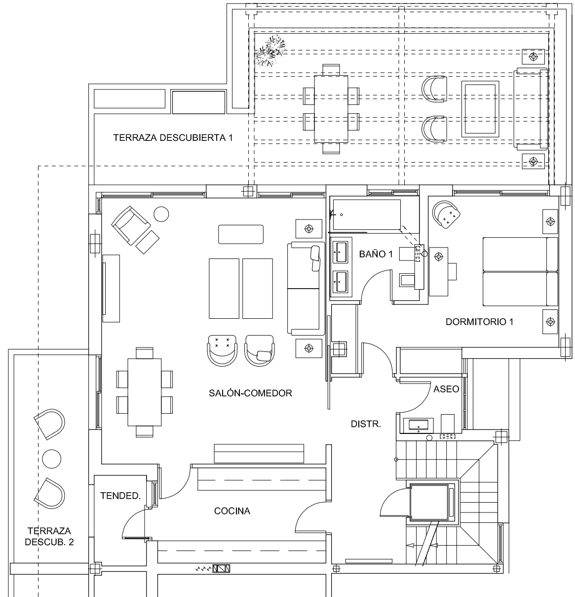
PLANTA ALTA
