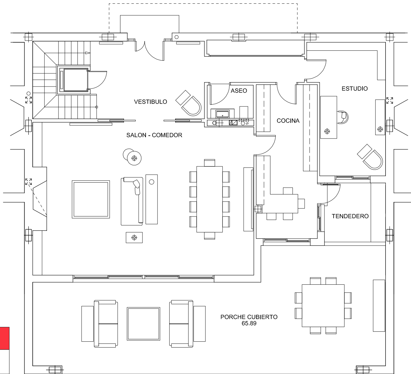
PLANTA BAJA
