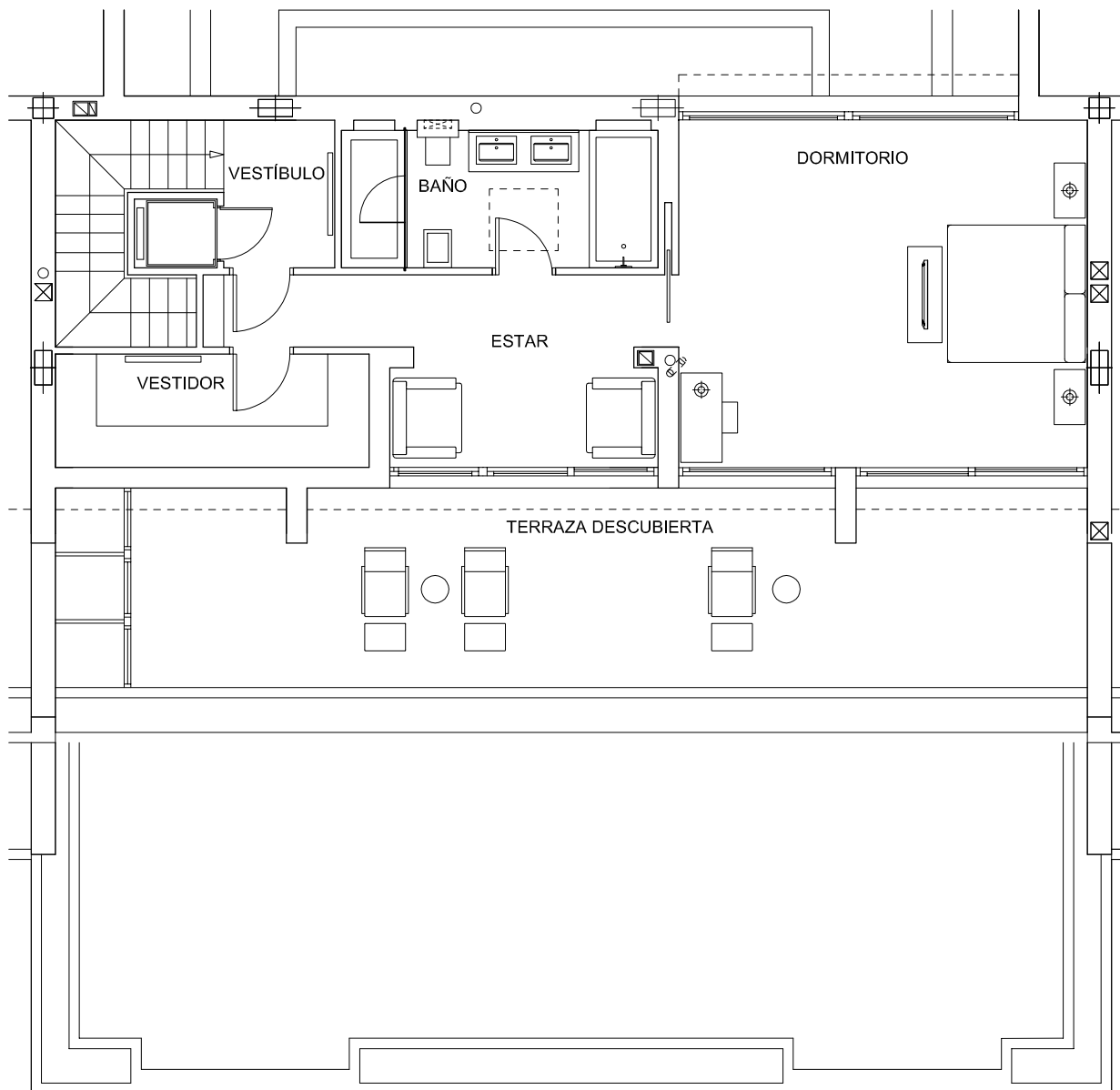
PLANTA SOLARIUM
