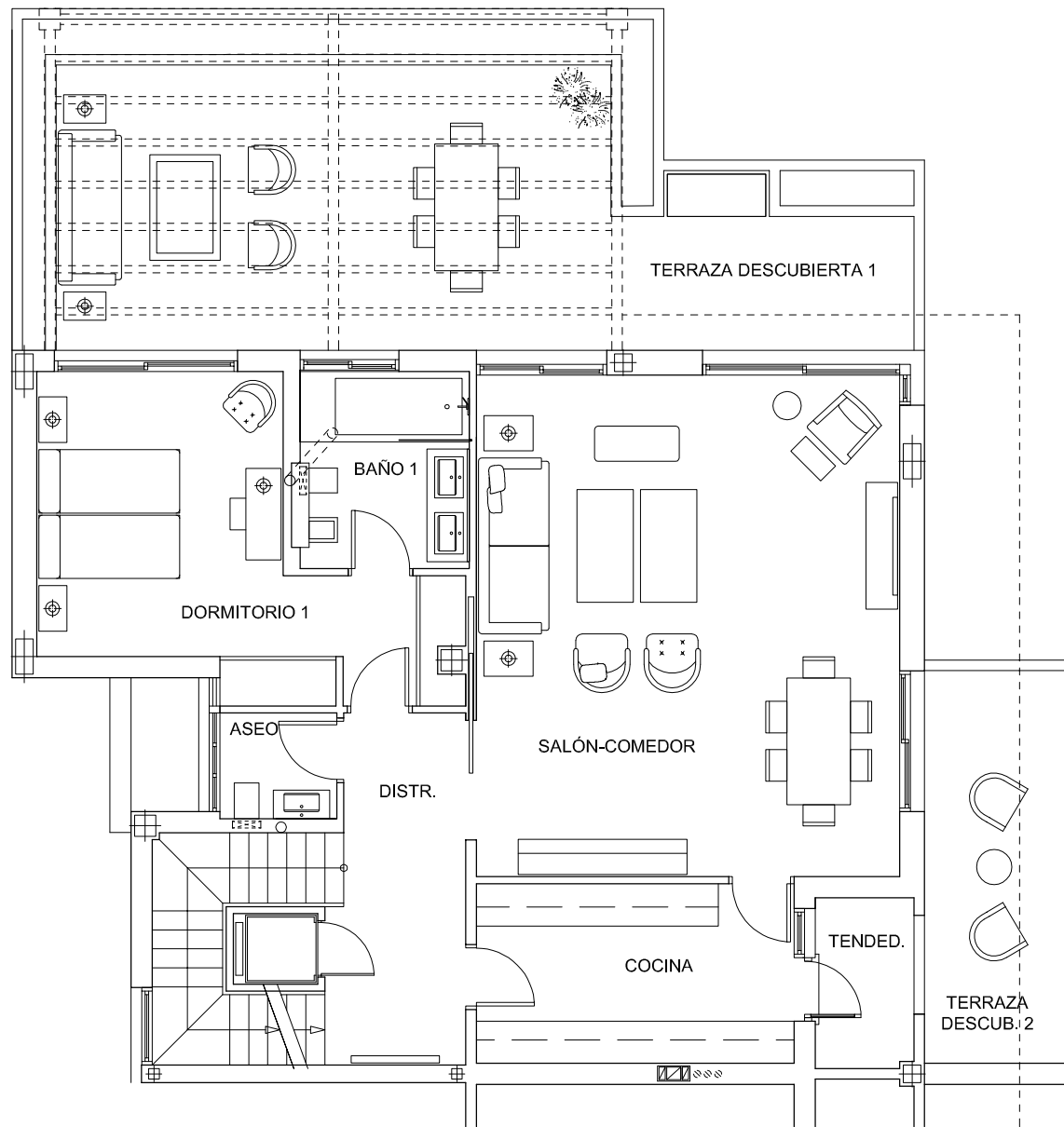
PLANTA ALTA
