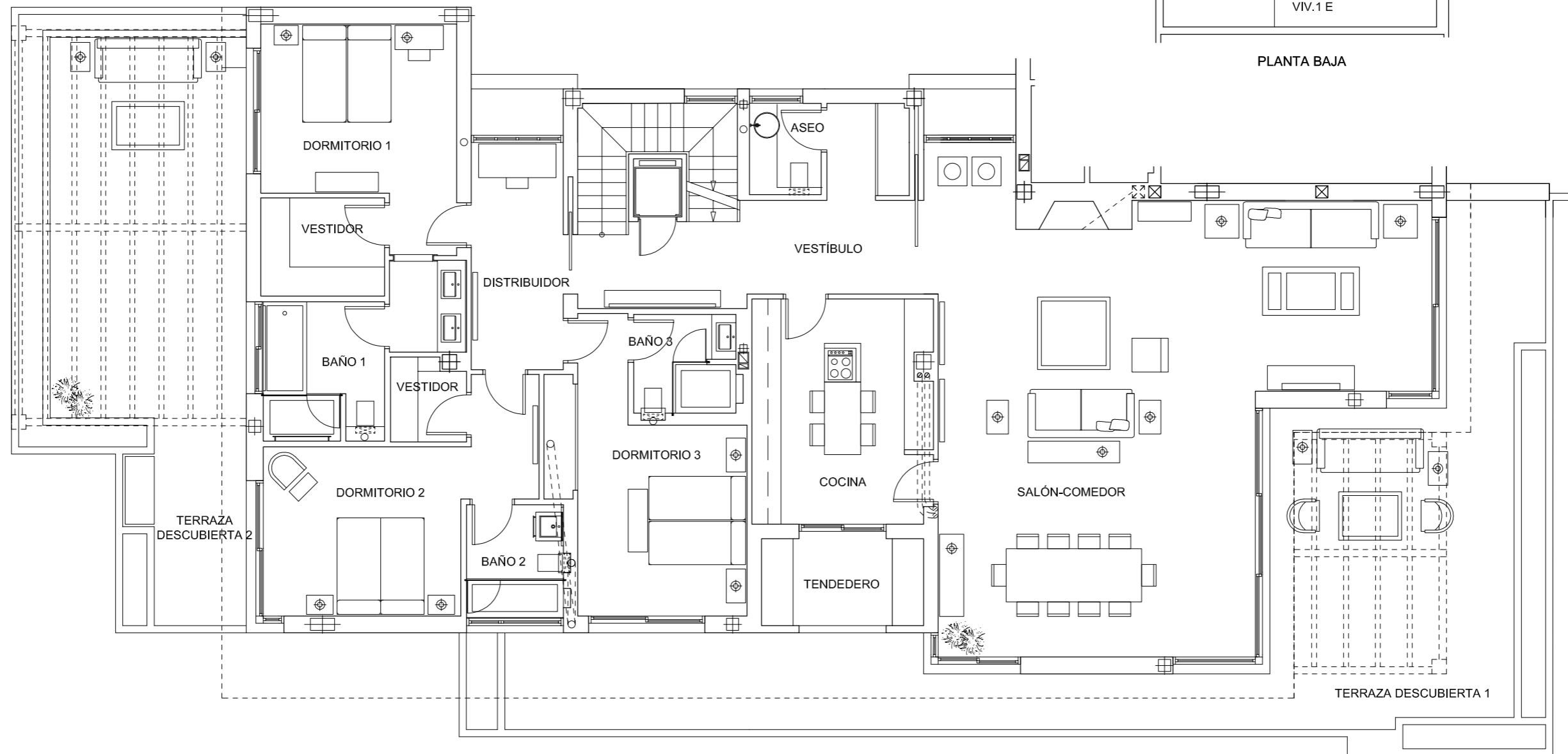
PLANTA ALTA
