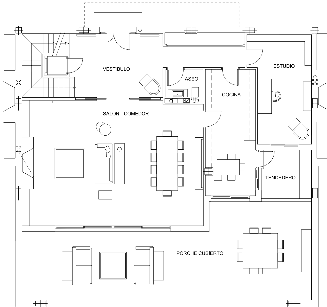
PLANTA BAJA
