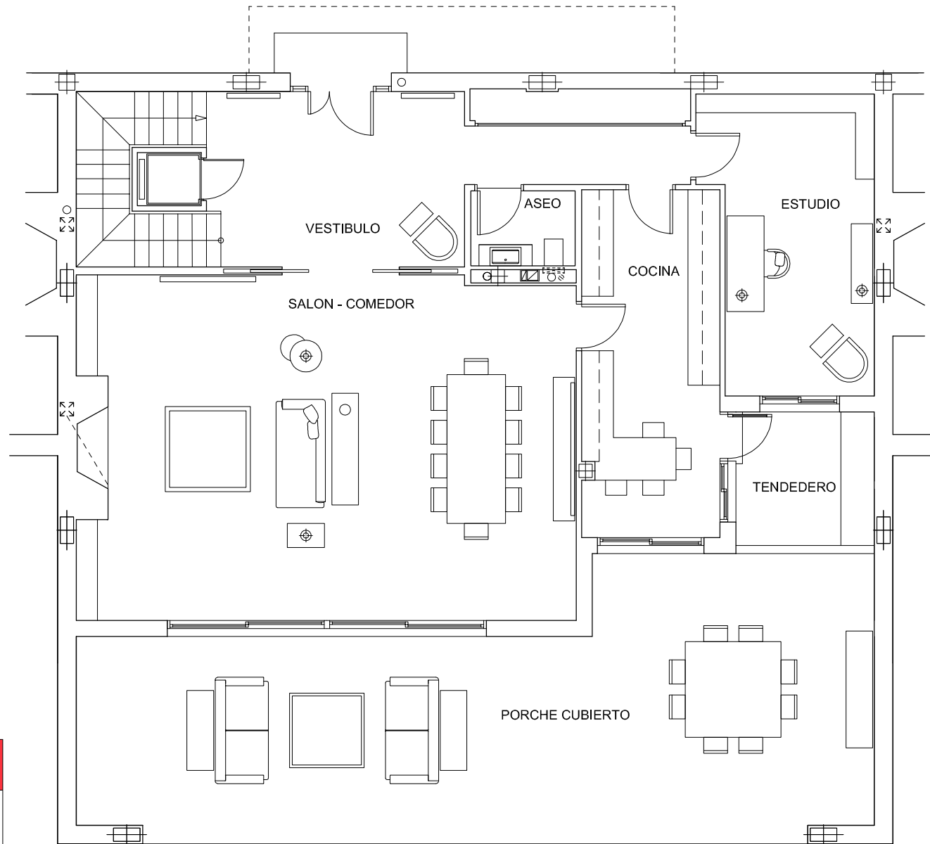
PLANTA BAJA
