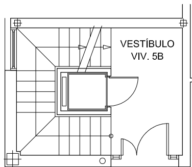
PLANTA BAJA
