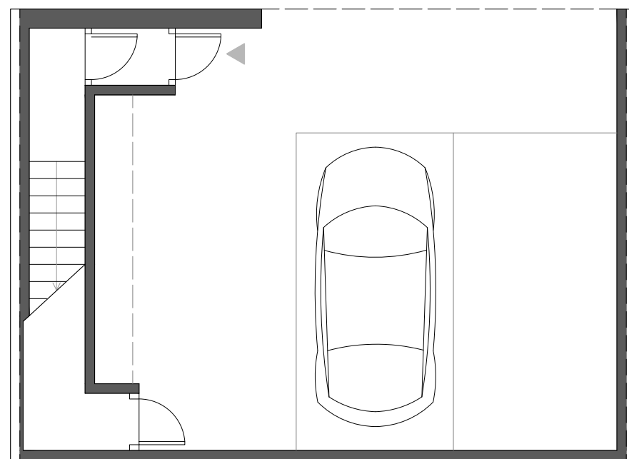
PLANTA SÓTANO
