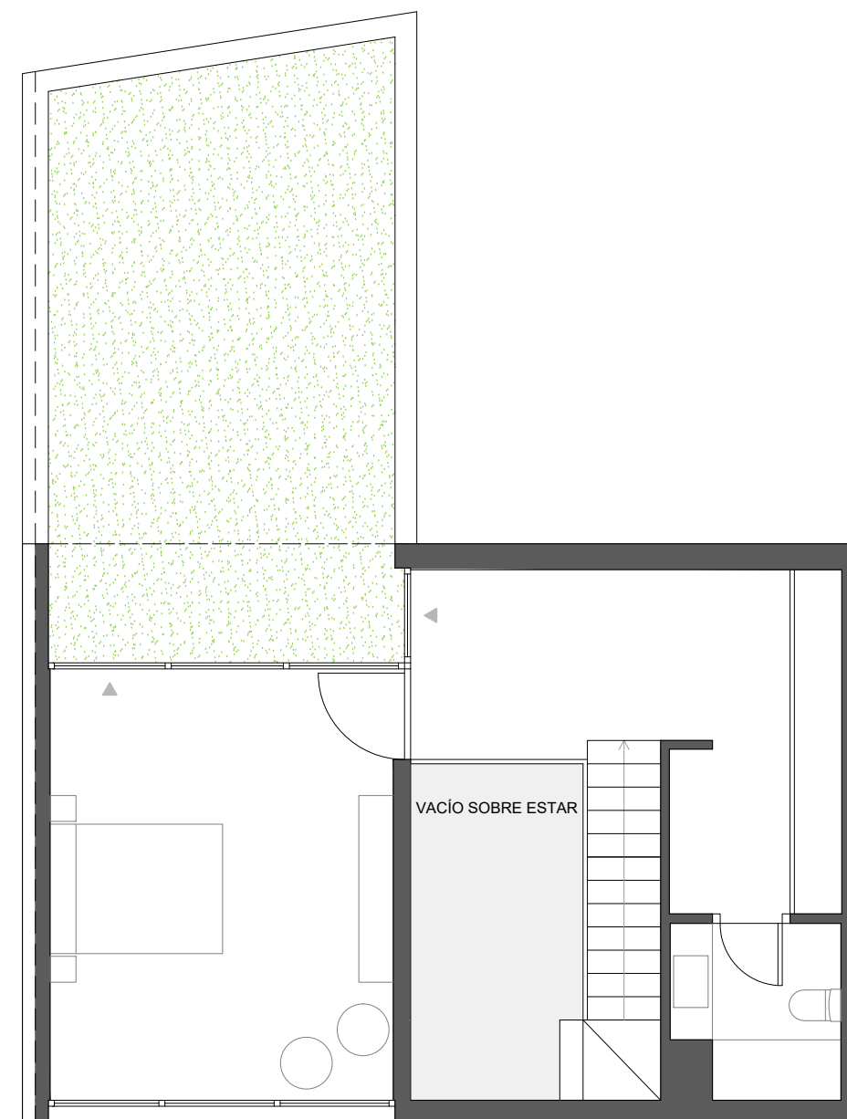
PLANTA SUPERIOR
