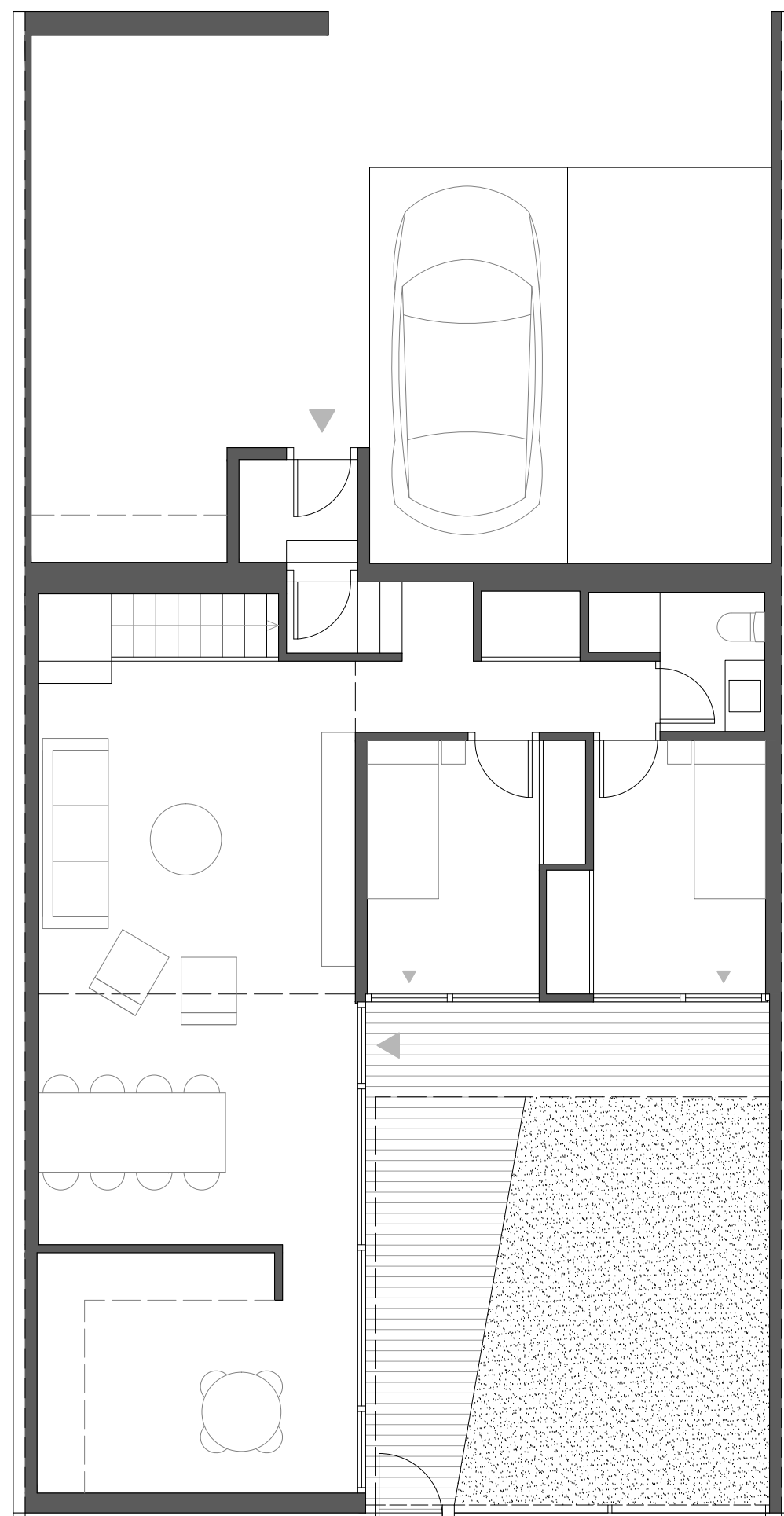
PLANTA INFERIOR
