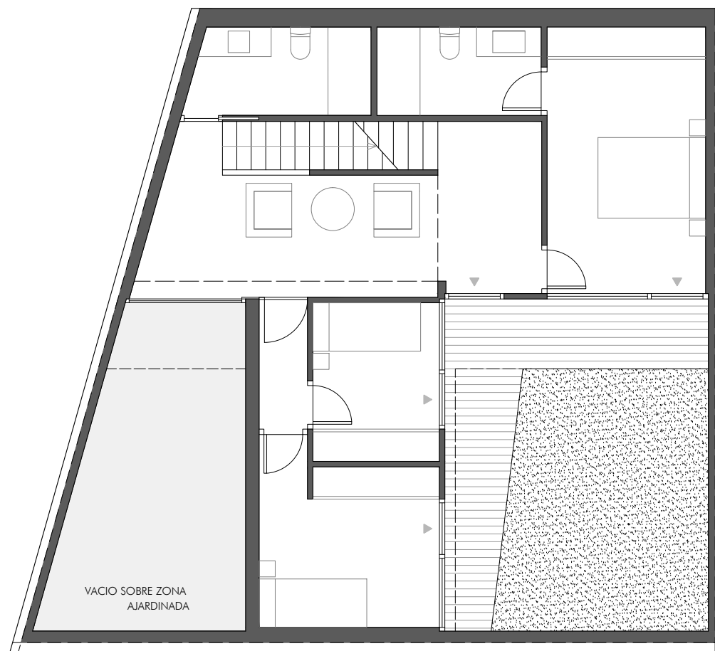
PLANTA INFERIOR
