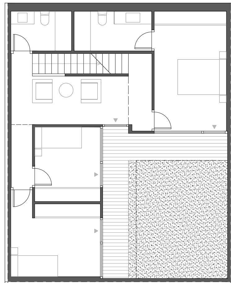
PLANTA INFERIOR
