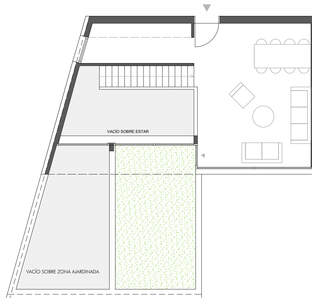
PLANTA SUPERIOR
