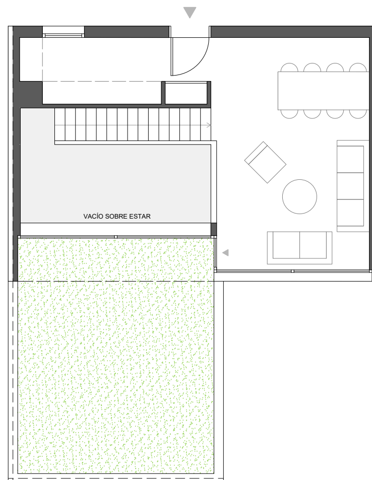
PLANTA SUPERIOR
