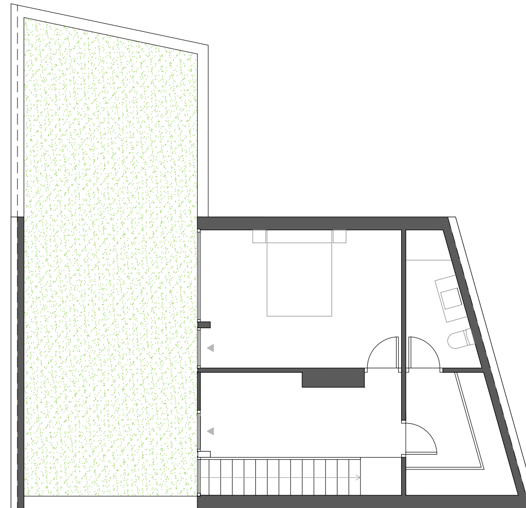
PLANTA SUPERIOR
