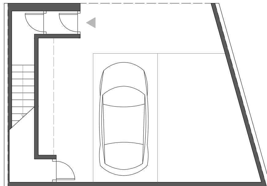
PLANTA SÓTANO
