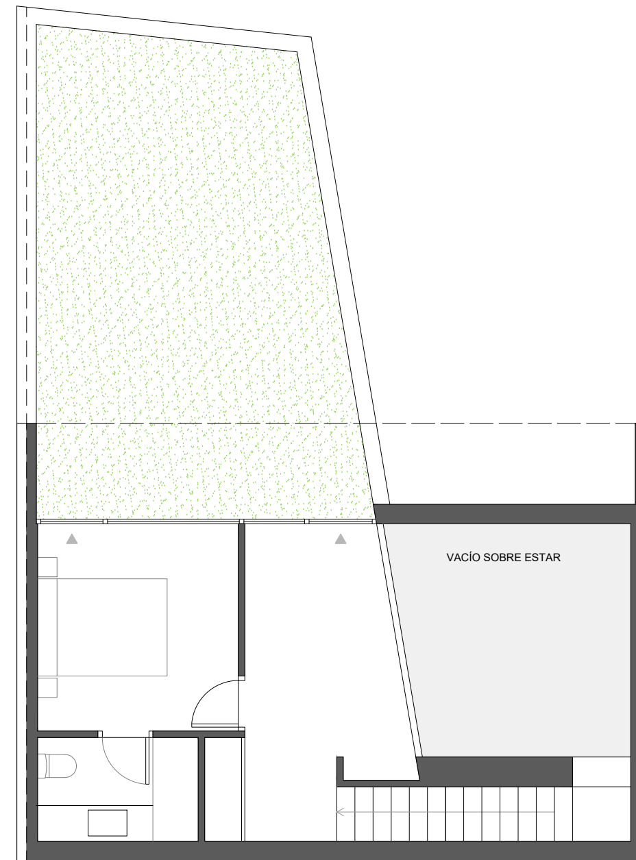
PLANTA SUPERIOR
