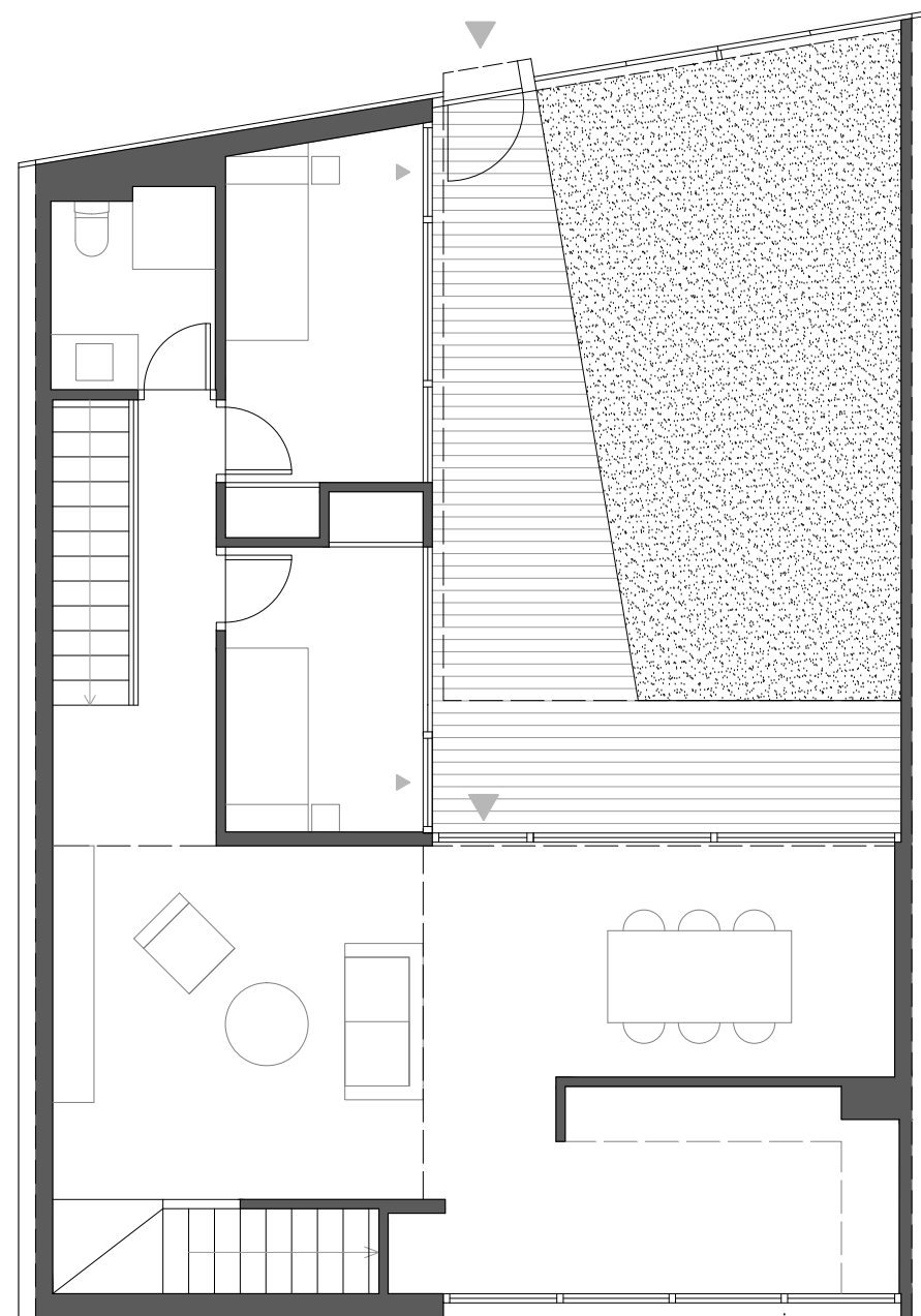
PLANTA INFERIOR
