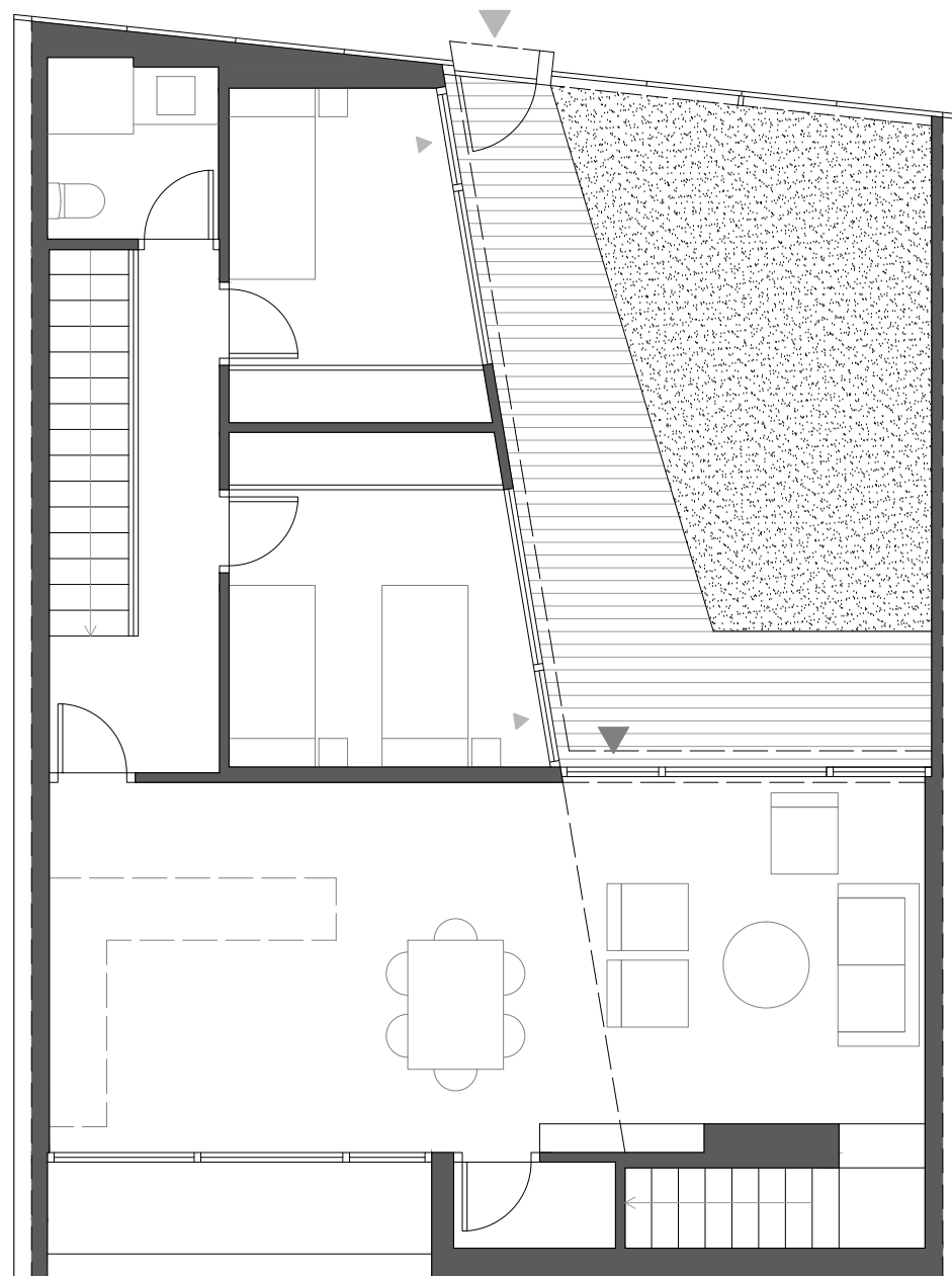
PLANTA INFERIOR
