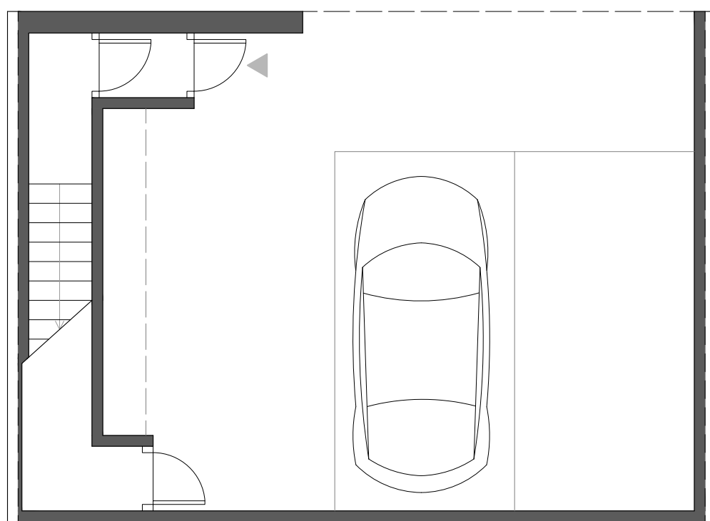
PLANTA SÓTANO
