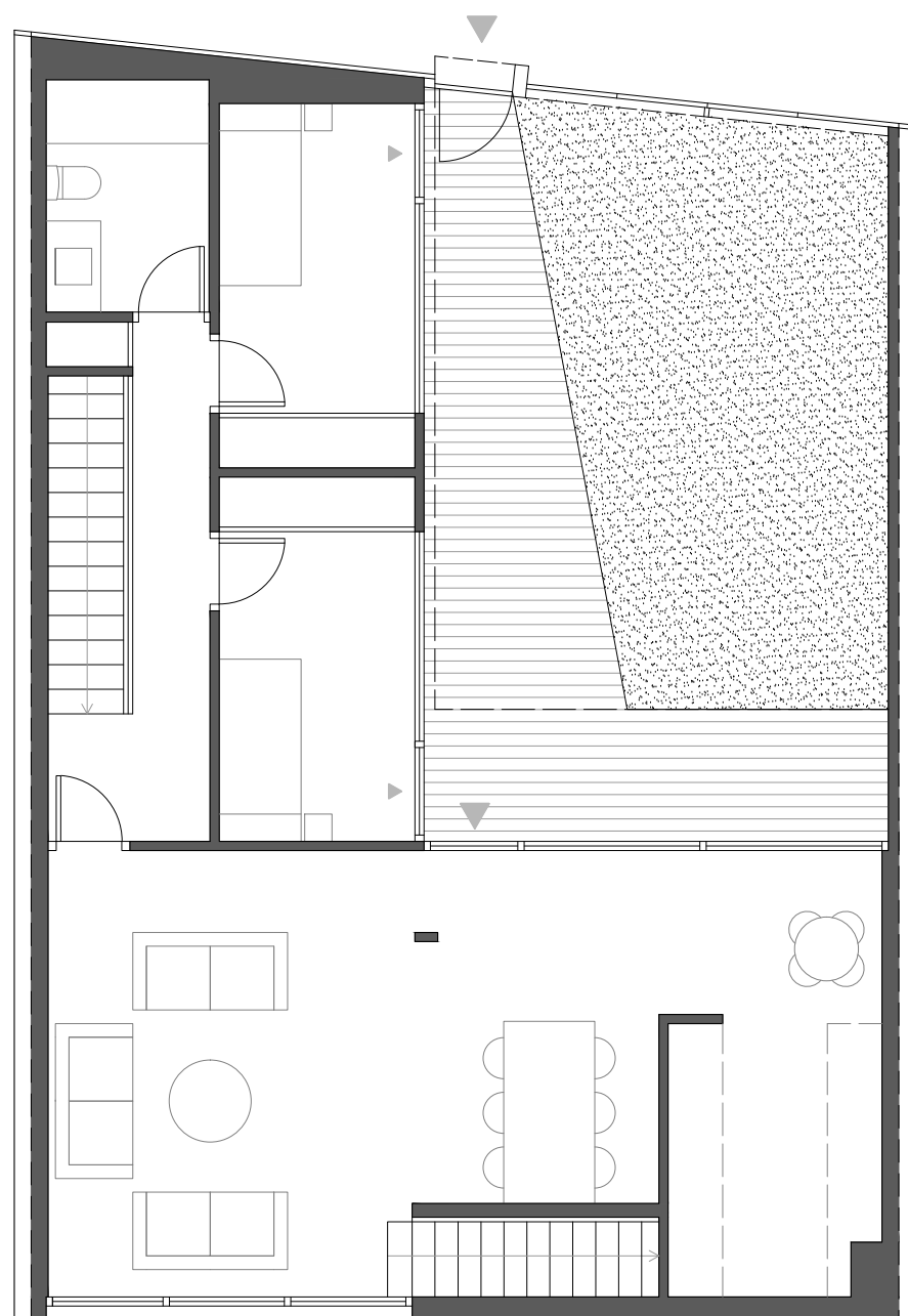
PLANTA INFERIOR
