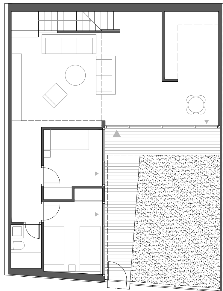
PLANTA INFERIOR
